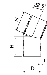
22.5°ベンド(22.5°マイター)
