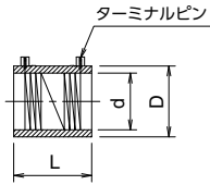
電気融着ソケット (EFS)
