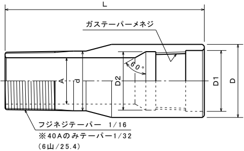
【上部ヘッド取合金具】
