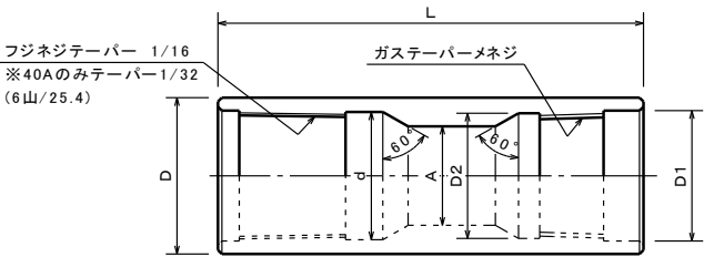
【下部水中ポンプ取合金具】
